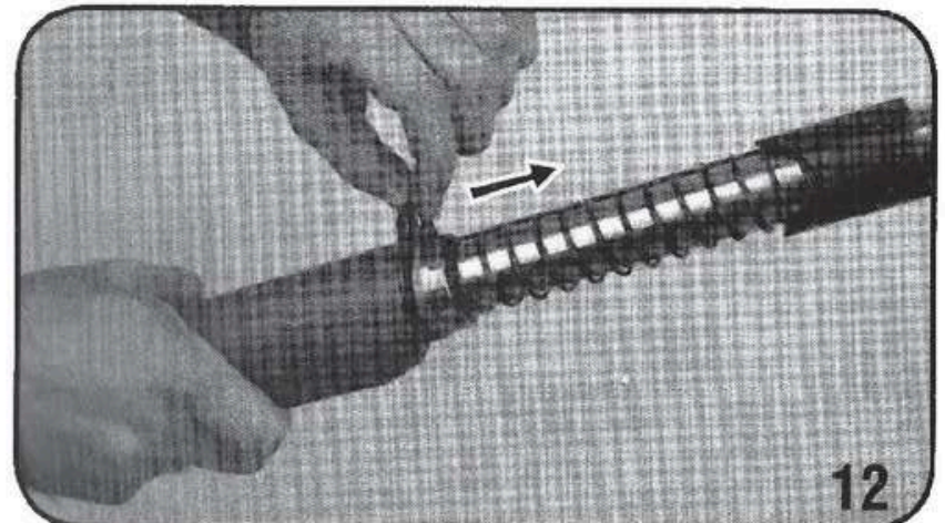
12. Remove the sling swivel nut.
